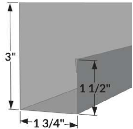
JT-3 - J Trim
