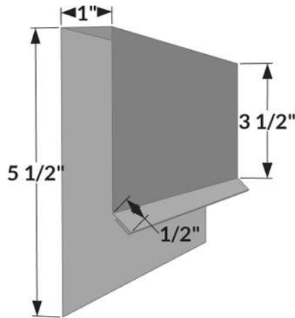
JT-5 - J Trim
