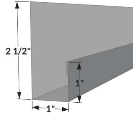
JT-3 - J Trim
