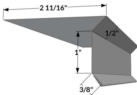
RK-1 - Rake Edge
