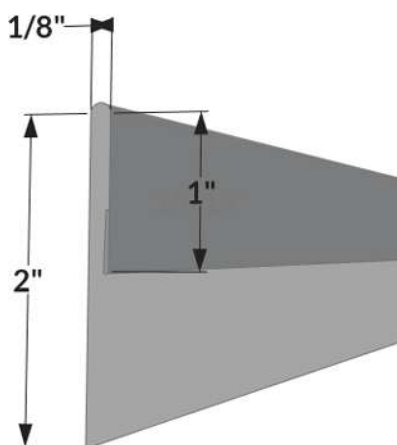
SLT-2 - Sill Trim
