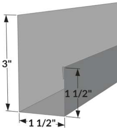
JT-4 - J Trim
