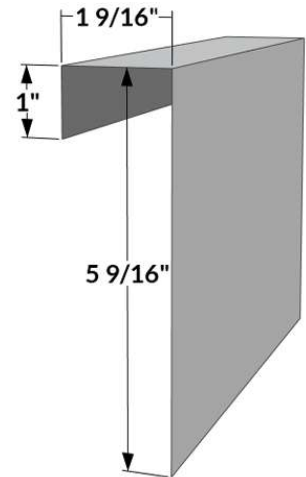
ODC-1 - O/H Door cap
