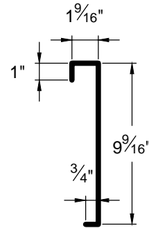
OVERHEAD DOOR CAP ODC-3
