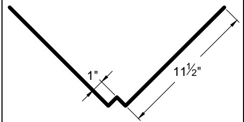
W-VALLEY VF-2
