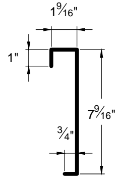
OVERHEAD DOOR CAP ODC-2
