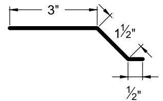
ROOF EDGE FLASHING RF-1
